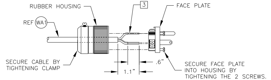
DETAIL B SCALE: 1:1
